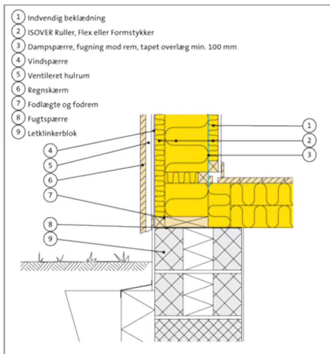
Fig. 410.50. Træskelet med ventileret regnskærm og kryd- slægtning - kælder.
