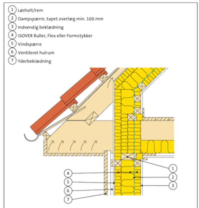
Fig. 410. 58. Træskelet med ventileret regnskærm og udvendig og indvendig krydslægtning - tagfod med varm skunk.
