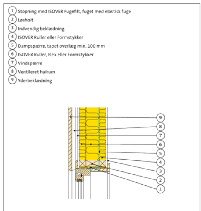
Fig. 410.64. Træskelet med ventileret regnskærm og udvendig og indvendig krydslægtning - overkant vindue.
