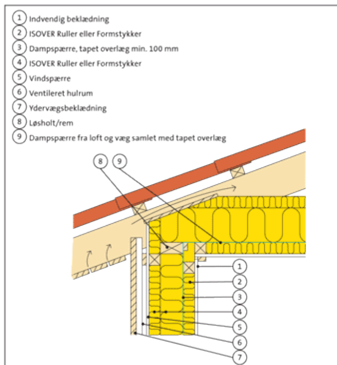
Fig. 410.56. Træskelet med ventileret regnskærm og udven- dig og indvendig krydslægtning - uudnyttet tagrum.
