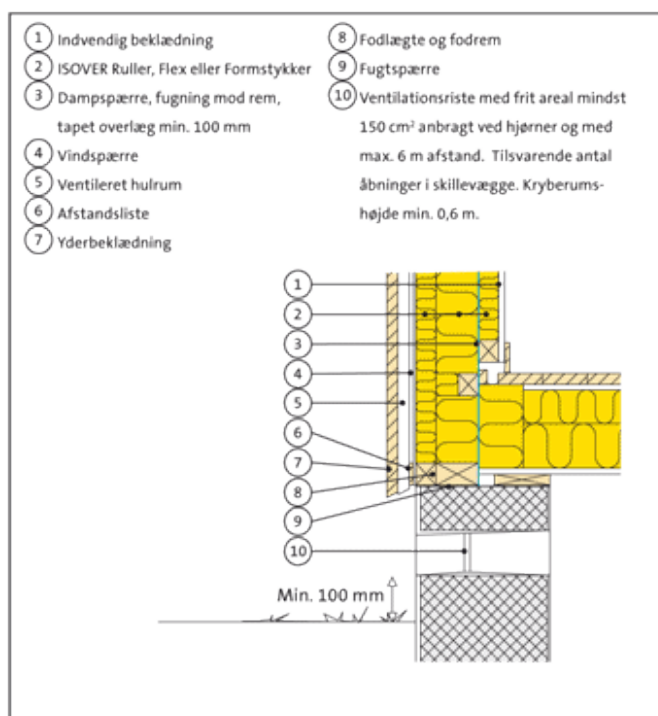
Fig. 410.51. Træskelet med ventileret regnskærm og kryd- slægtning - krybekælder.
