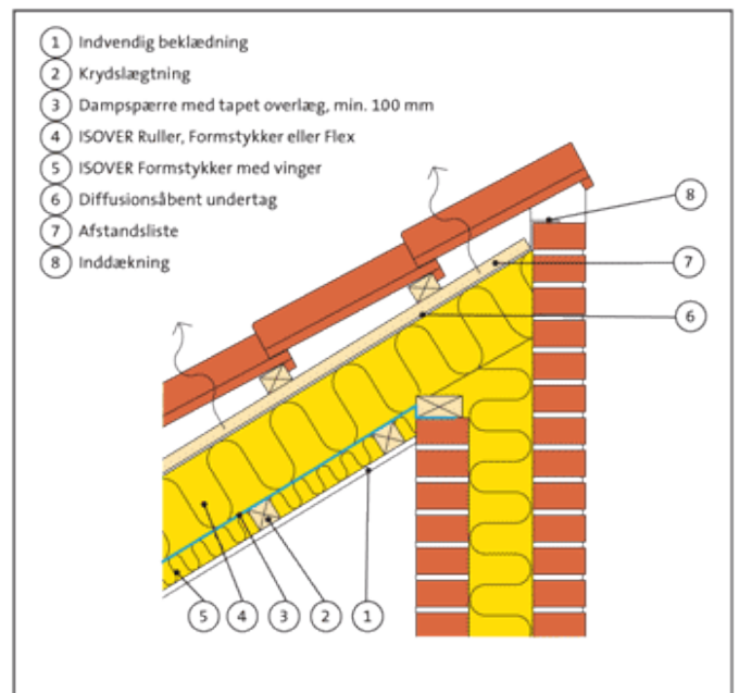
Fig. 310.47. Bjælkespær. Isolering og diffusionsåbent undertag.
