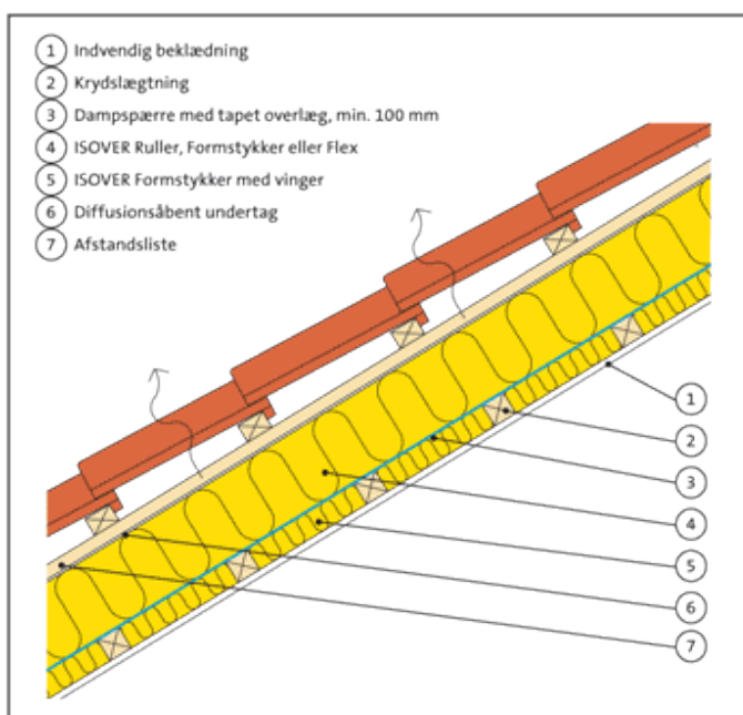
Fig. 310.48. Bjælkespær. Tegltag med diffusionsåbent undertag.
