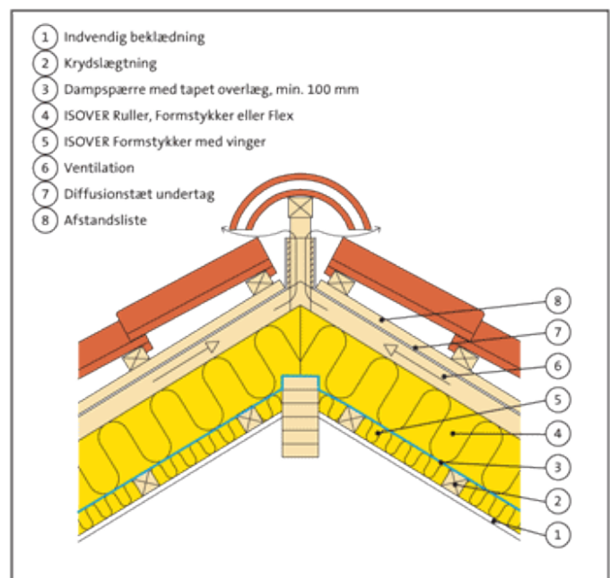
Fig. 310.49. Detaljer ved kipdrager.
